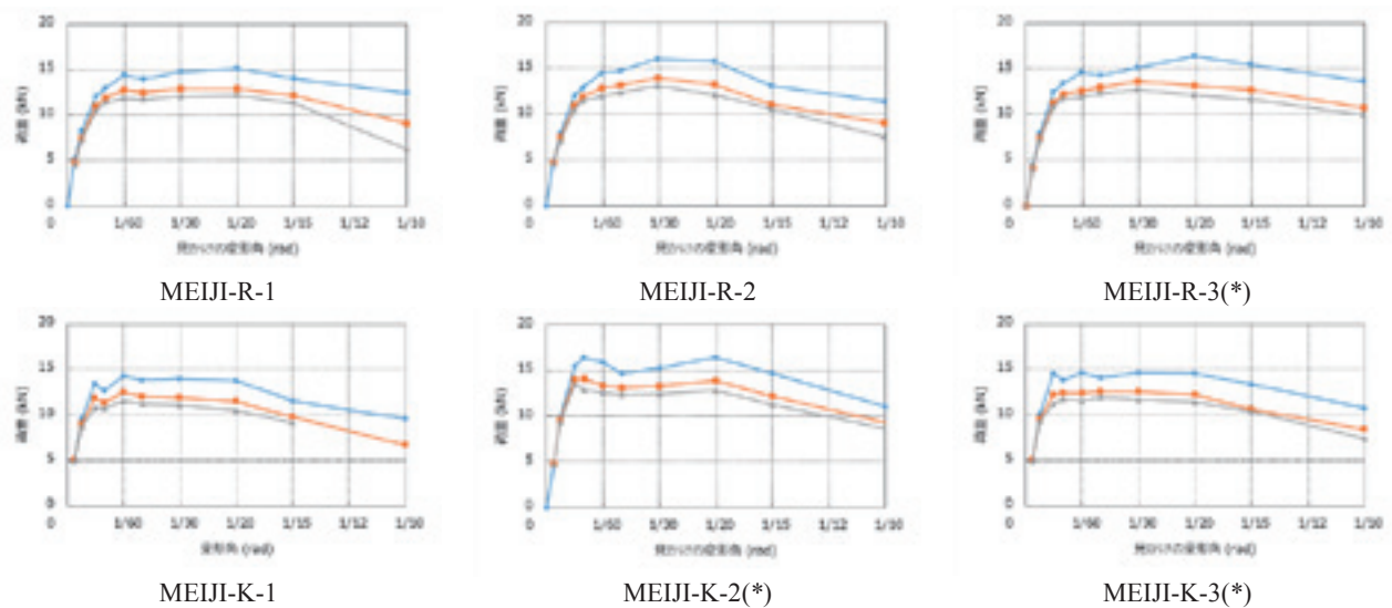
図 5 包絡線（青色線は 1 回目、赤色線は 2 回目、灰色線は 3 回目の繰り返しを示す）
