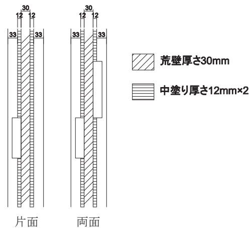
図 2 壁厚さは 54mm
