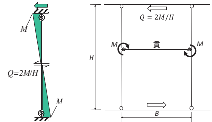
図 7 長ほぞ仕口、貫仕口のモーメント抵抗によるせん断力
